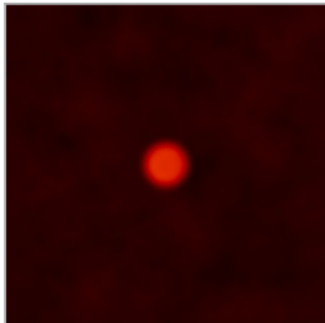
TrapezoidDisk2DKernel
