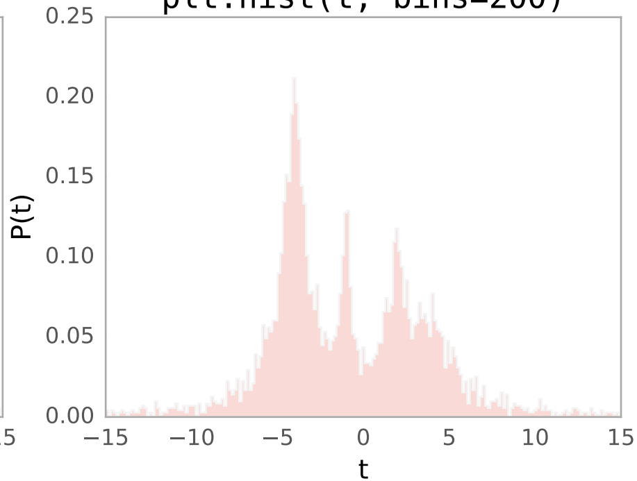
plt.hist(t, bins=200)
