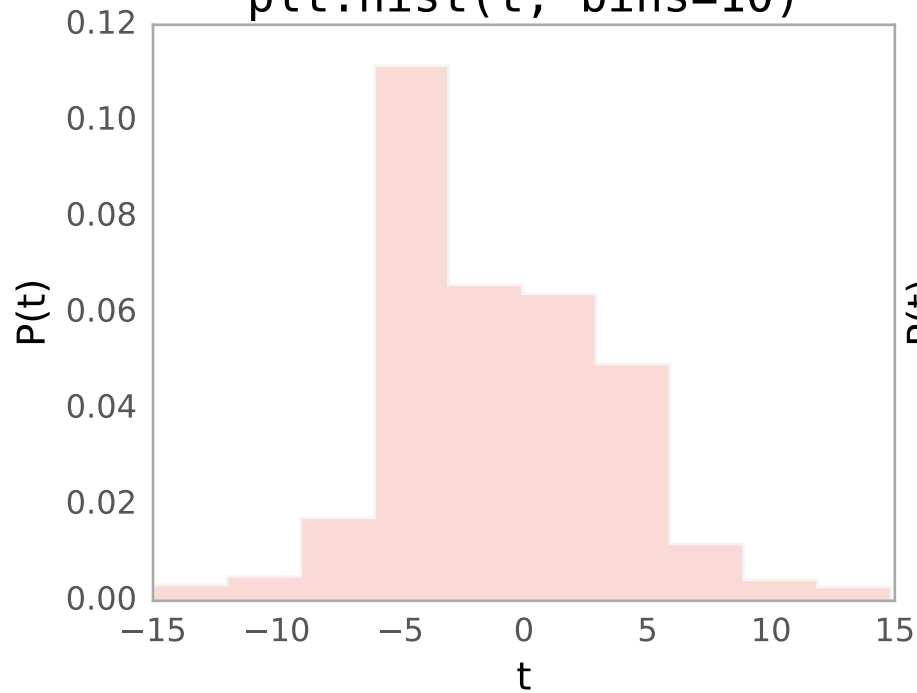
plt.hist(t, bins=10)
